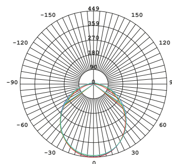
CURVA FOTOMETRICA
